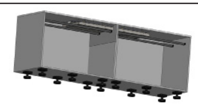
ג2.3: התקן 2 סטים של סרגלי התמיכות של פיט קוקינג בהתאם להוראות ההתקנה.
