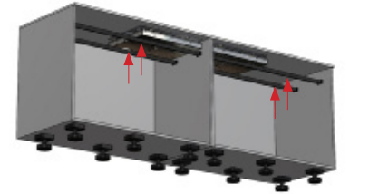
ב3: התקן 2 סטים של סרגלי התמיכות של פיט קוקינג בהתאם להוראות ההתקנה.
