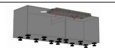
ג2.1: מקם את דגם פיט קוקינג בתוך הארון דרך החיתוך הקדמי מתחת למשטח העבודה. זהירות! יש לשים לב לגובה החיתוך: 150 מ"מ למערכת עם מתגים עליונים/200 מ"מ לדגם עם מתגים קדמיים, מתחתית משטח העבודה.
