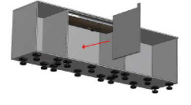
ג2: התקן את דגם הפיט קוקינג בהתאם להוראות ההתקנה התקניים ולאחר מכן החזר את המחיצה האמצעית עם המגרעת.
