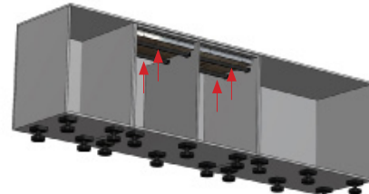
ג3: התקן 2 סטים של סרגלי התמיכות של פיט קוקינג בהתאם להוראות ההתקנה.
