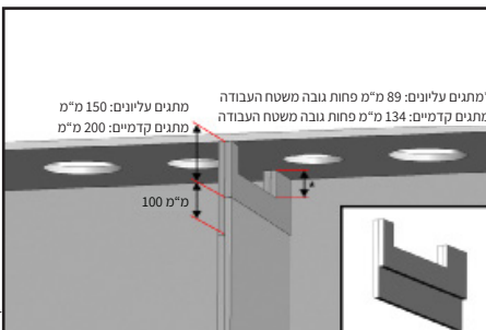
אפשרות ג': שני ארונות
