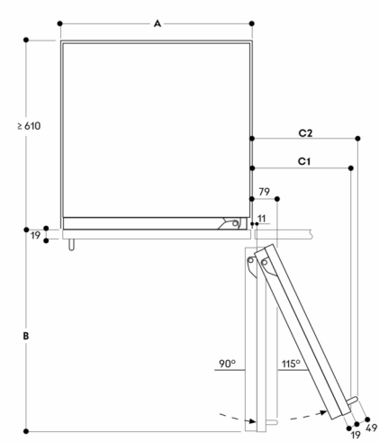
Wall clearance RVB / RVC / RVF / RVW
