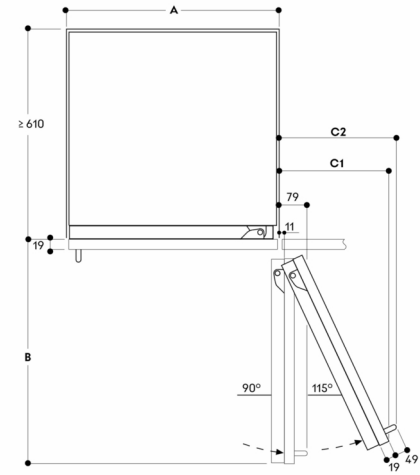
Wall clearance RVB / RVC / RVF / RVW
