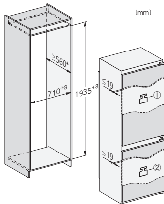
KFN7934D, XXL built-in, Einbau
