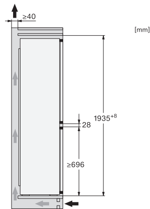
KFN7934D, XXL built-in, Seitenansicht
